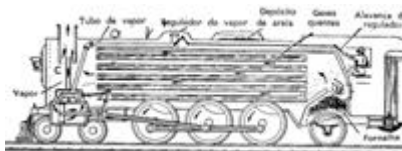
Locomotiva a vapor
