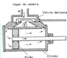
Máquina a vapor
